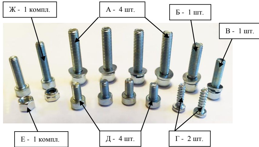
Комплект крепежа и пояснительная схема его установки
